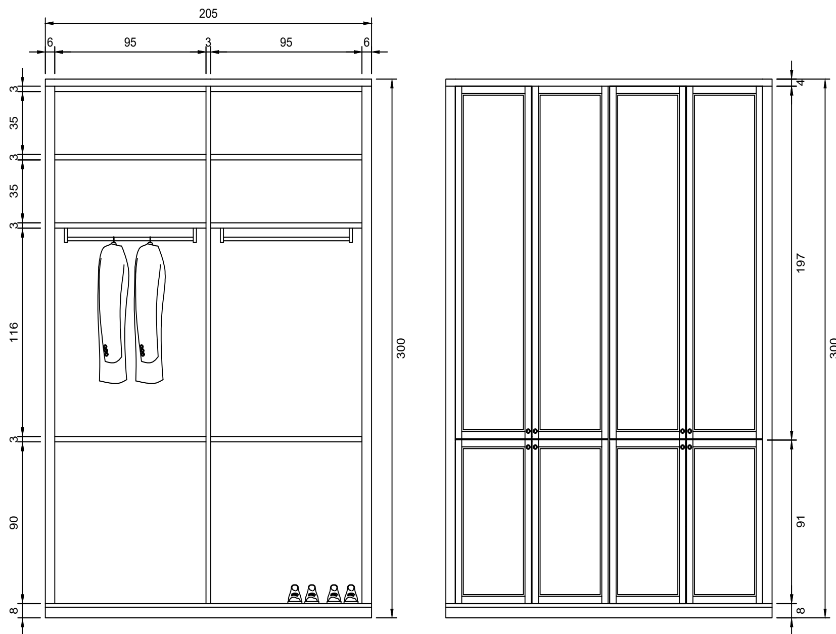
Prospetto frontale:
