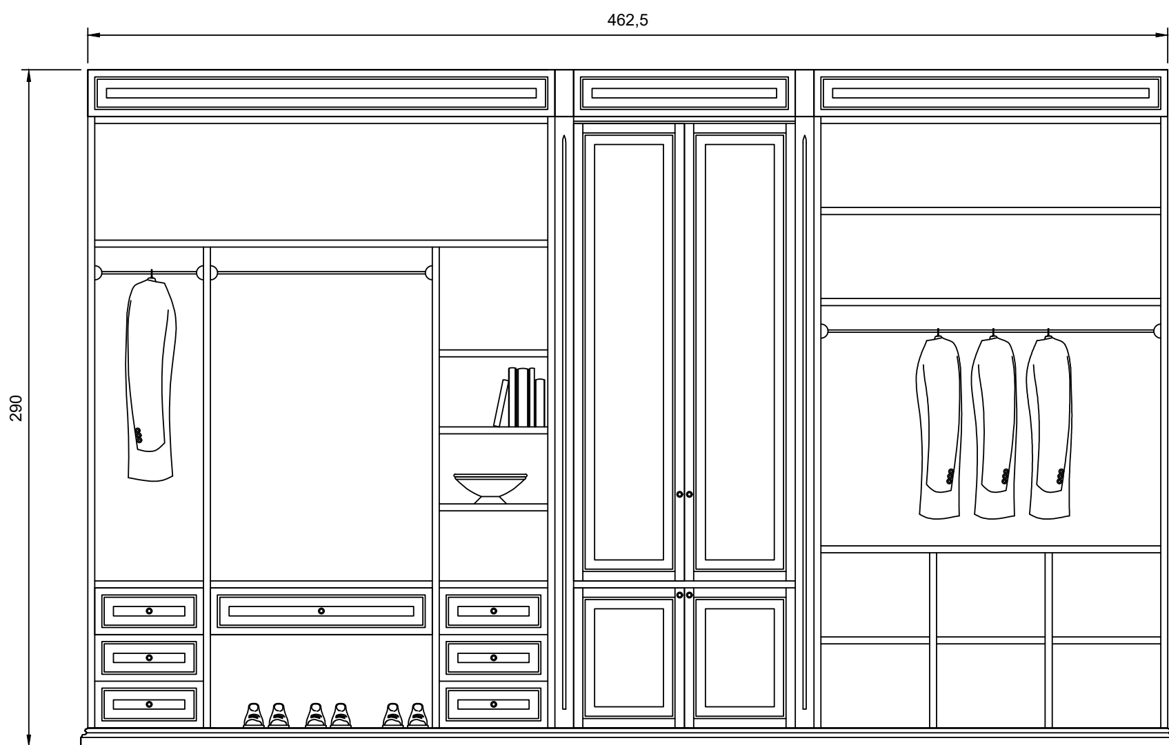
Prospetto frontale:
